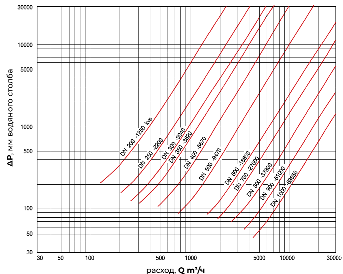
Диаграмма потери давления на обратном клапане
