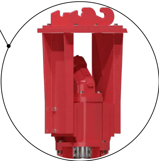
НАСОС HERACLES® С ГИДРОМОТОРОМ
