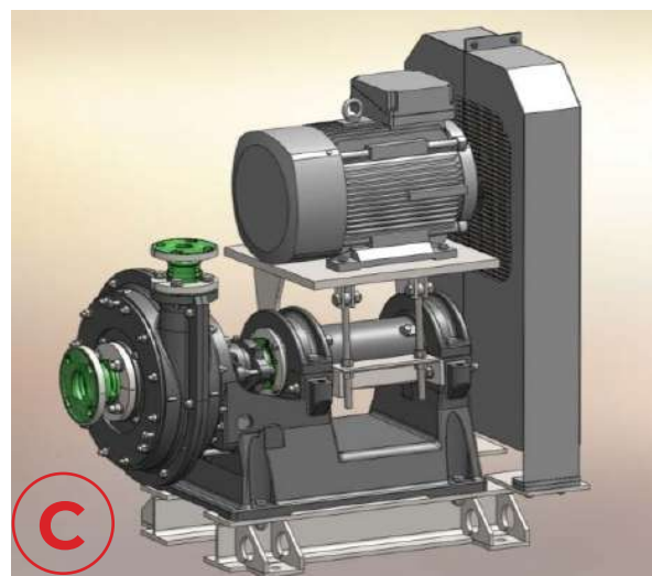
Привод насоса через клиновидный ремень, электродвигатель расположен над подшипниковым узлом насоса
