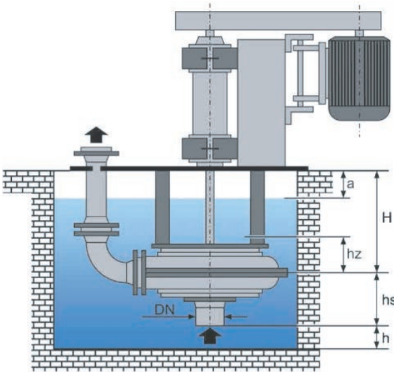
Мокрая установка V300 (Максимальная высота всасывания hs = 2500 мм)
